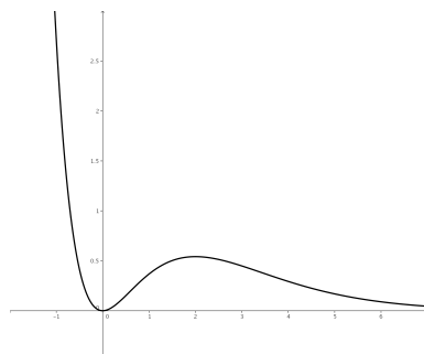
Figura 1.11: Representación gráfica de la función f(x) = x^2 \cdot e^{-x}
