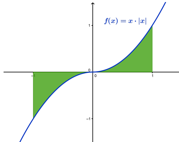
Figura 1.39: Representación gráfica del área buscada.
