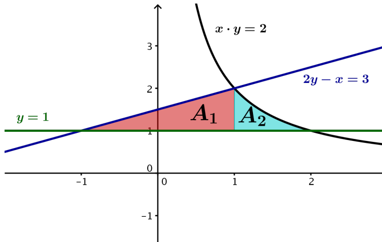
Figura 1.47: Representación de la región requerida
