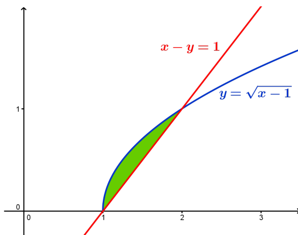
Figura 1.31: Representación detallada del área buscada
