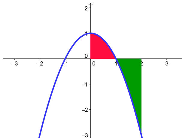
Figura 1.48: Representación gráfica de la región pedida
