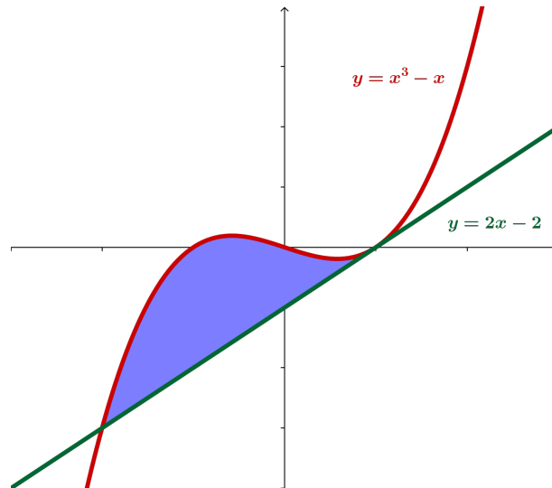
Figura 1.22: Representación detallada del área buscada
