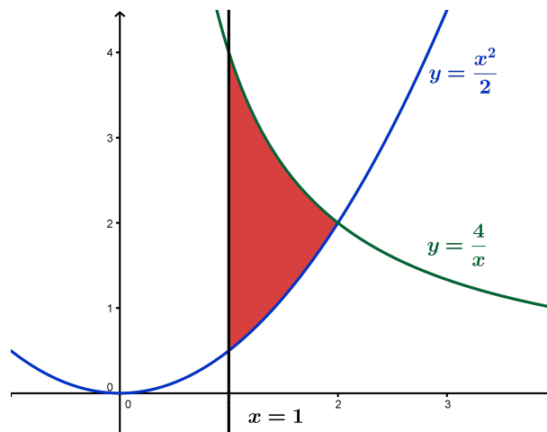
Figura 1.41: Representación gráfica de las funciones \frac{x^2}{2} y \frac{4}{x}
