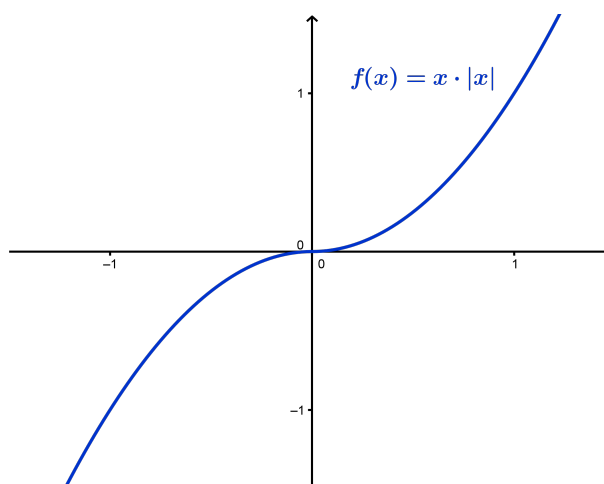
Figura 1.38: Representación gráfica de la función f(x) = x \cdot |x| .
