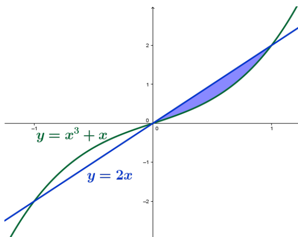
Figura 1.28: Visión gráfica del problema
