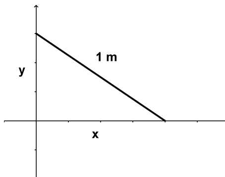
Figura 1.8: Visión gráfica del problema
