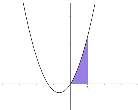
Figura 1.21: Representación detallada del área buscada
