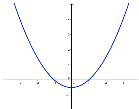
Figura 1.33: Representación gráfica de la función f(x) = \frac{1}{2}x^2 - \frac{1}{2}
