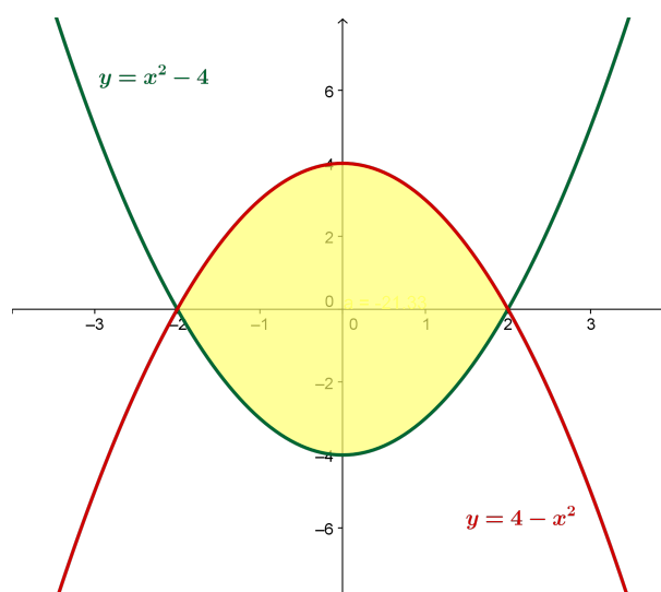
Figura 1.23: Representación gráfica de la región pedida.
