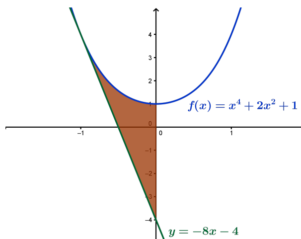
Figura 1.42: Representación del área requerida
