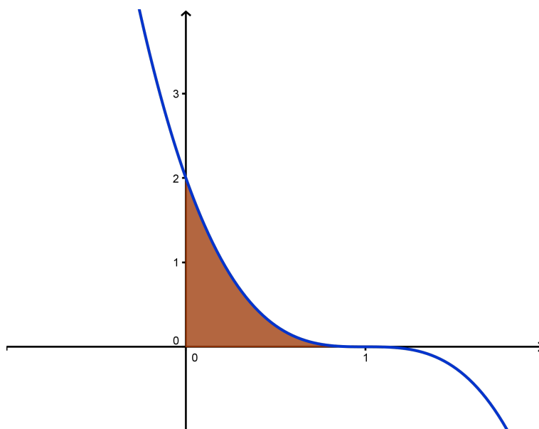
Figura 1.45: Representación de la región requerida
