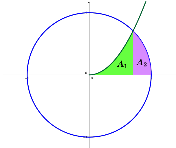
Figura 1.20: Representación detallada del área buscada
