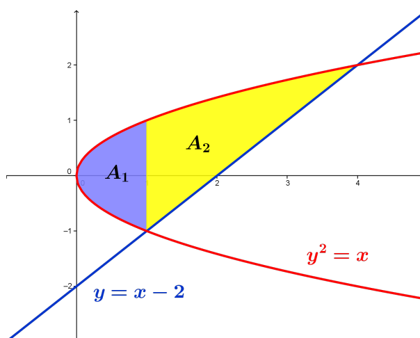
Figura 1.25: Representación gráfica de la región pedida.
