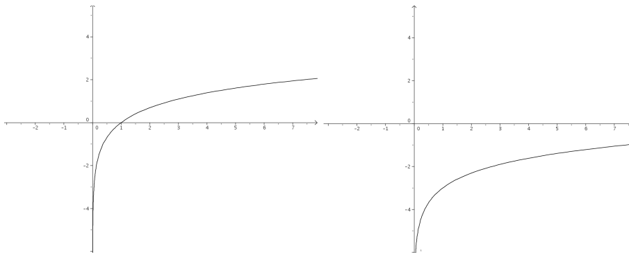
Figura 1.27: Gráfica de y = \ln x y de y = \ln x - 3
