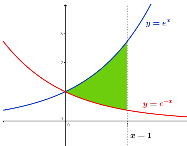
Figura 1.30: Área encerrada por las exponenciales y x=1 .
