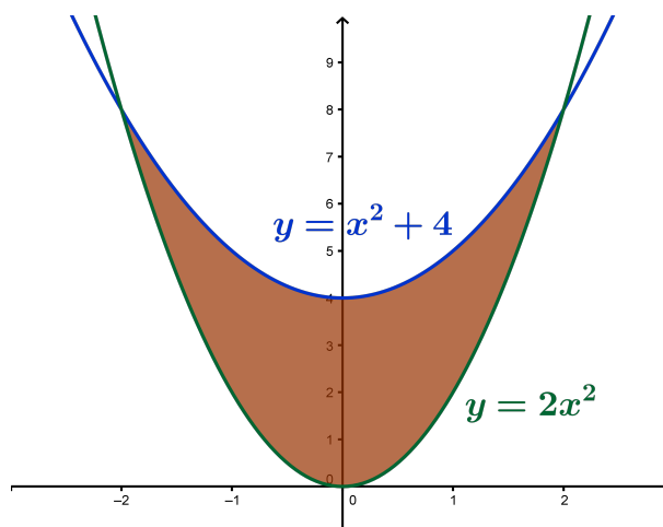
Figura 1.43: Representación de la región requerida
